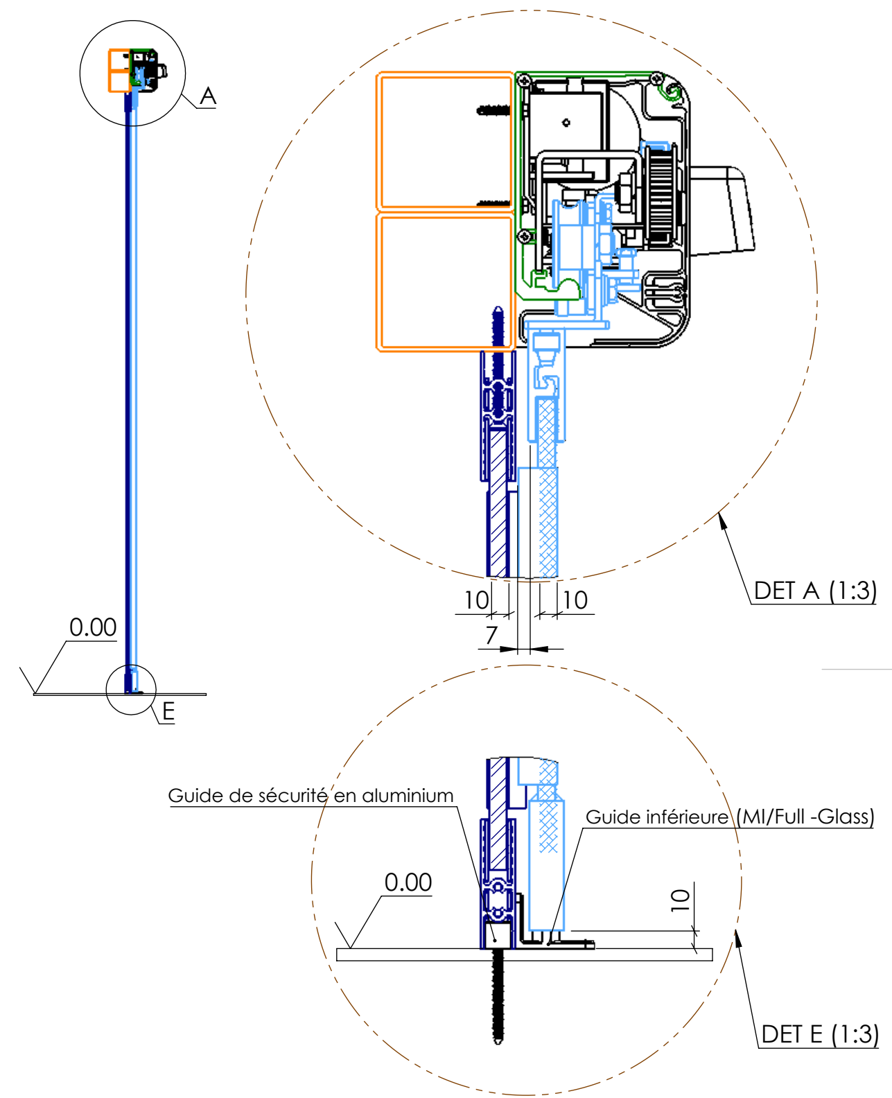
Coupe verticale: Profil de la poutre
