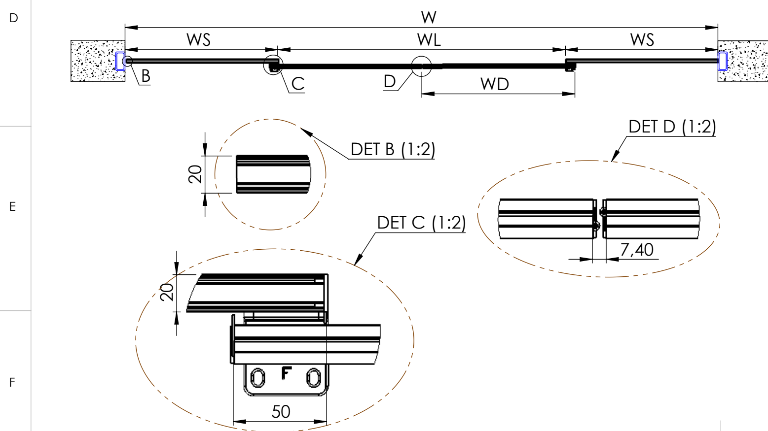
Sección horizontal:
