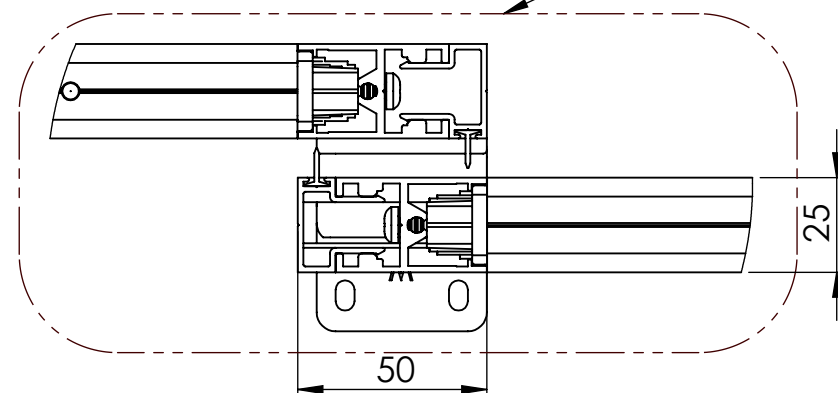
DET C (1:2)
