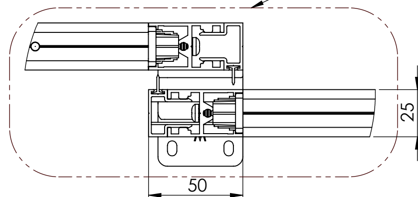
DET C (1:2)
