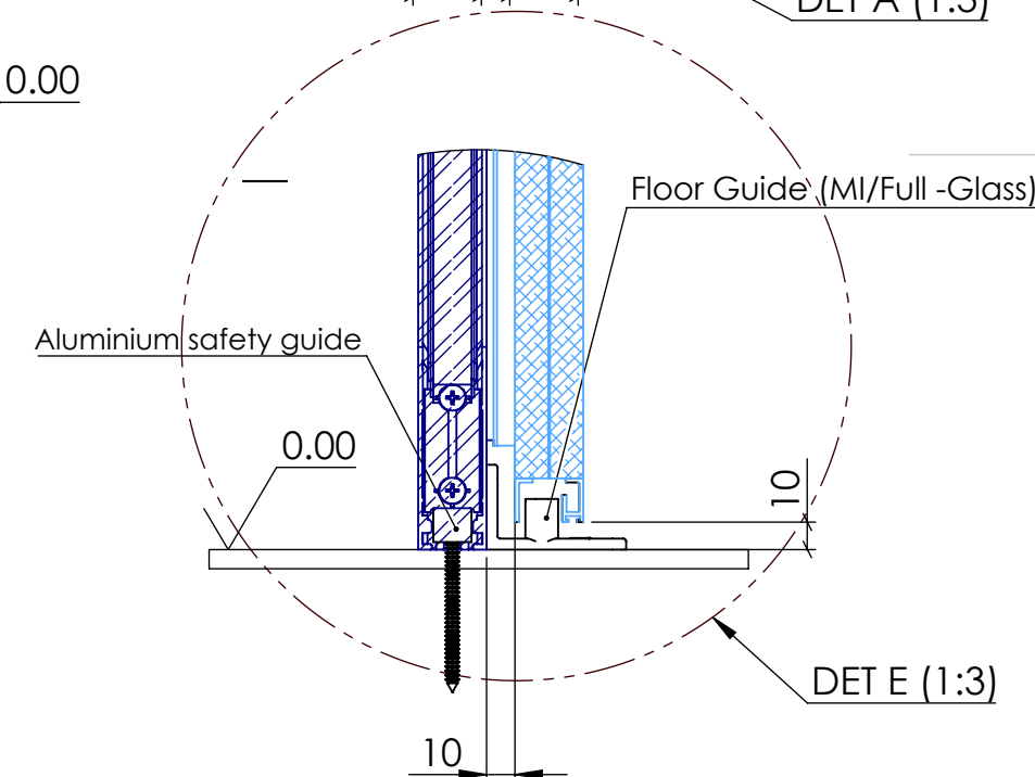
DET A (1:3)
