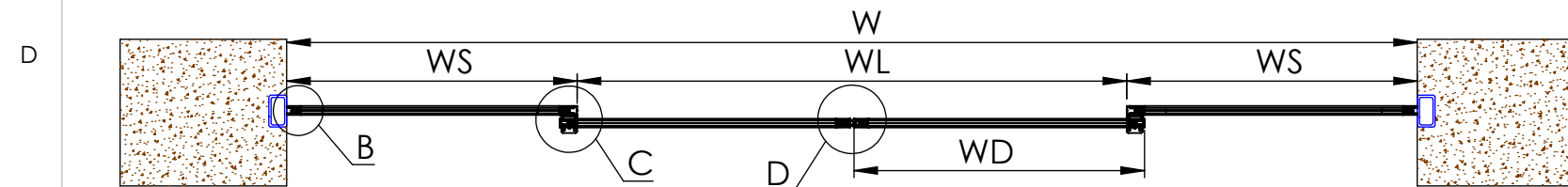
Sección horizontal:
