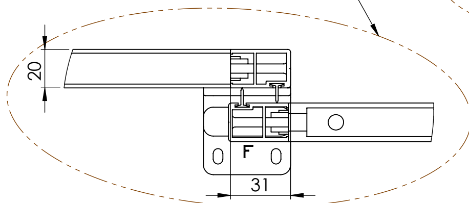
DET C (1:2)
