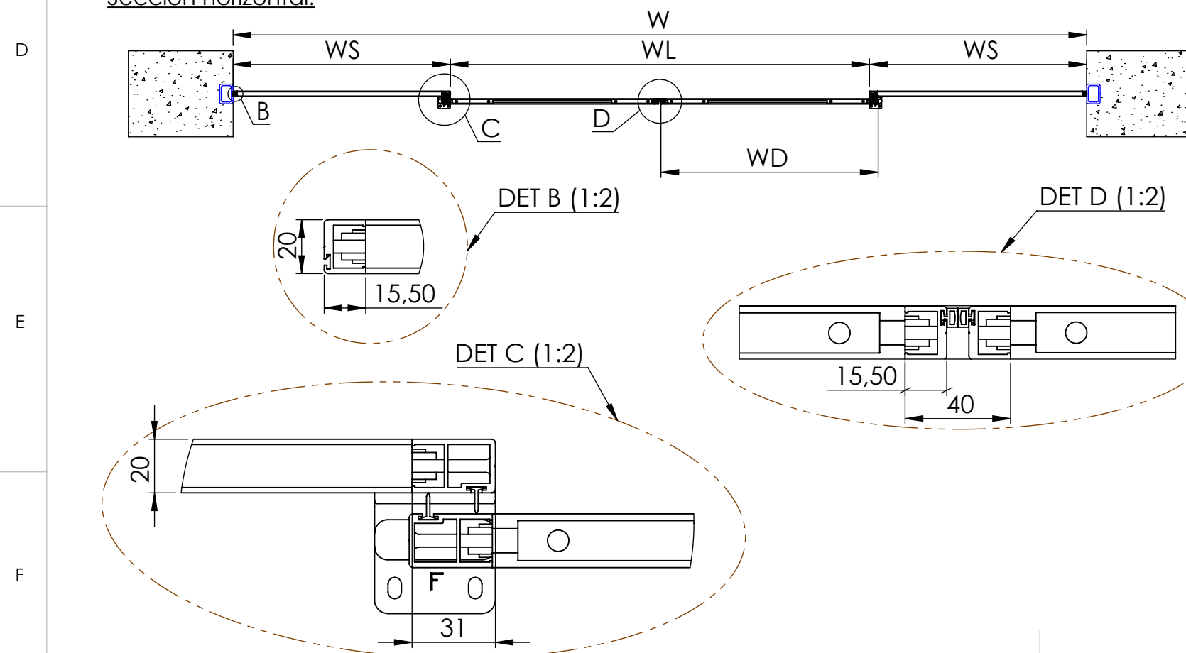
Sección horizontal:
