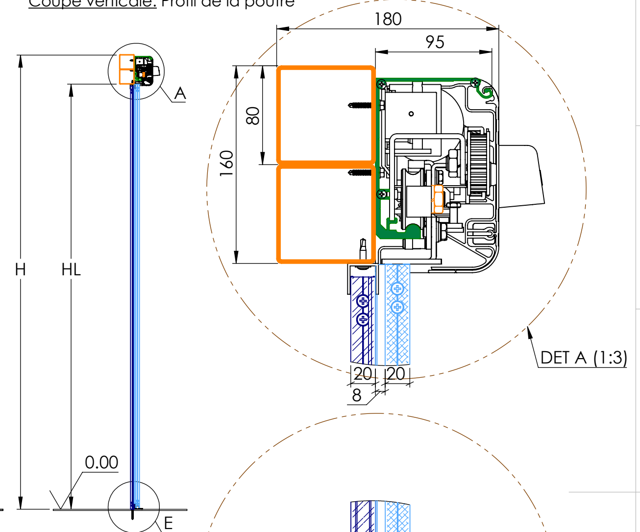
Coupe verticale: Profil de la poutre
