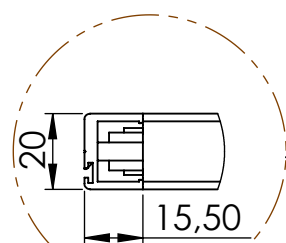
DET B (1:2)
